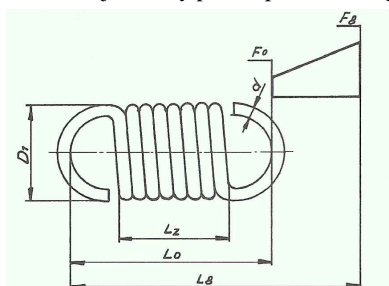
Příklad objednávky pružin podle katalogu: Tažná pružina T d x D 1 x L 0 x z
